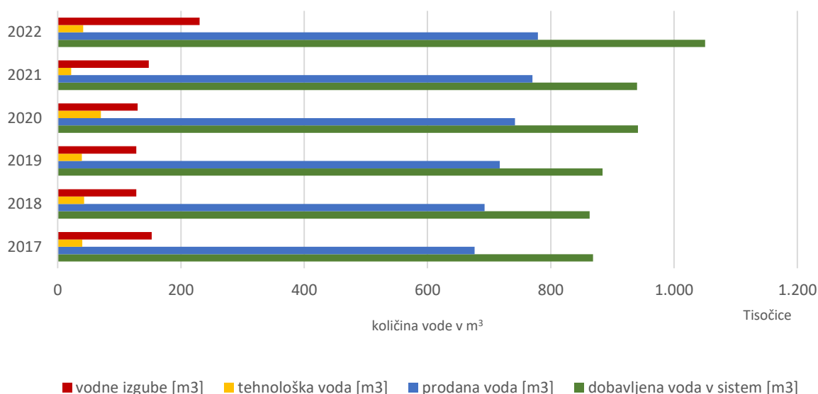
Graf 12: Prikaz vodne bilance na vseh vodovodnih sistemih skupaj 2017 - 2022
